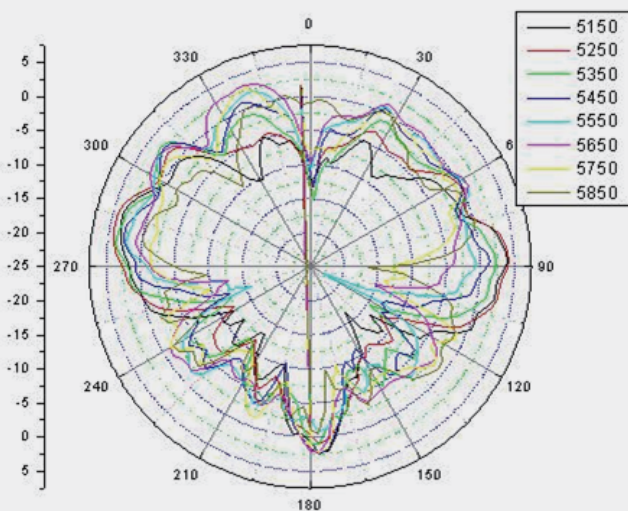
5G (PHI=0)
