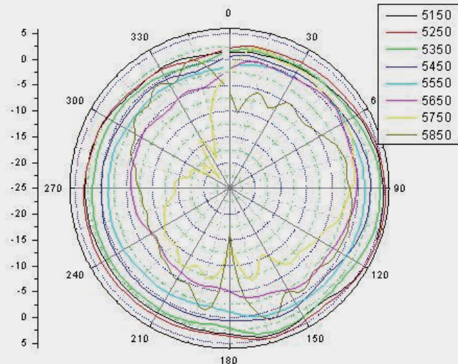
5G (PHI=90)
